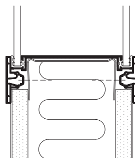
Gips-glassamling - lodret snit
