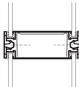
Glassamling - lodret snit
