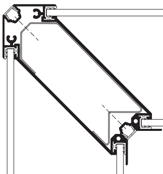
90° hjørne
